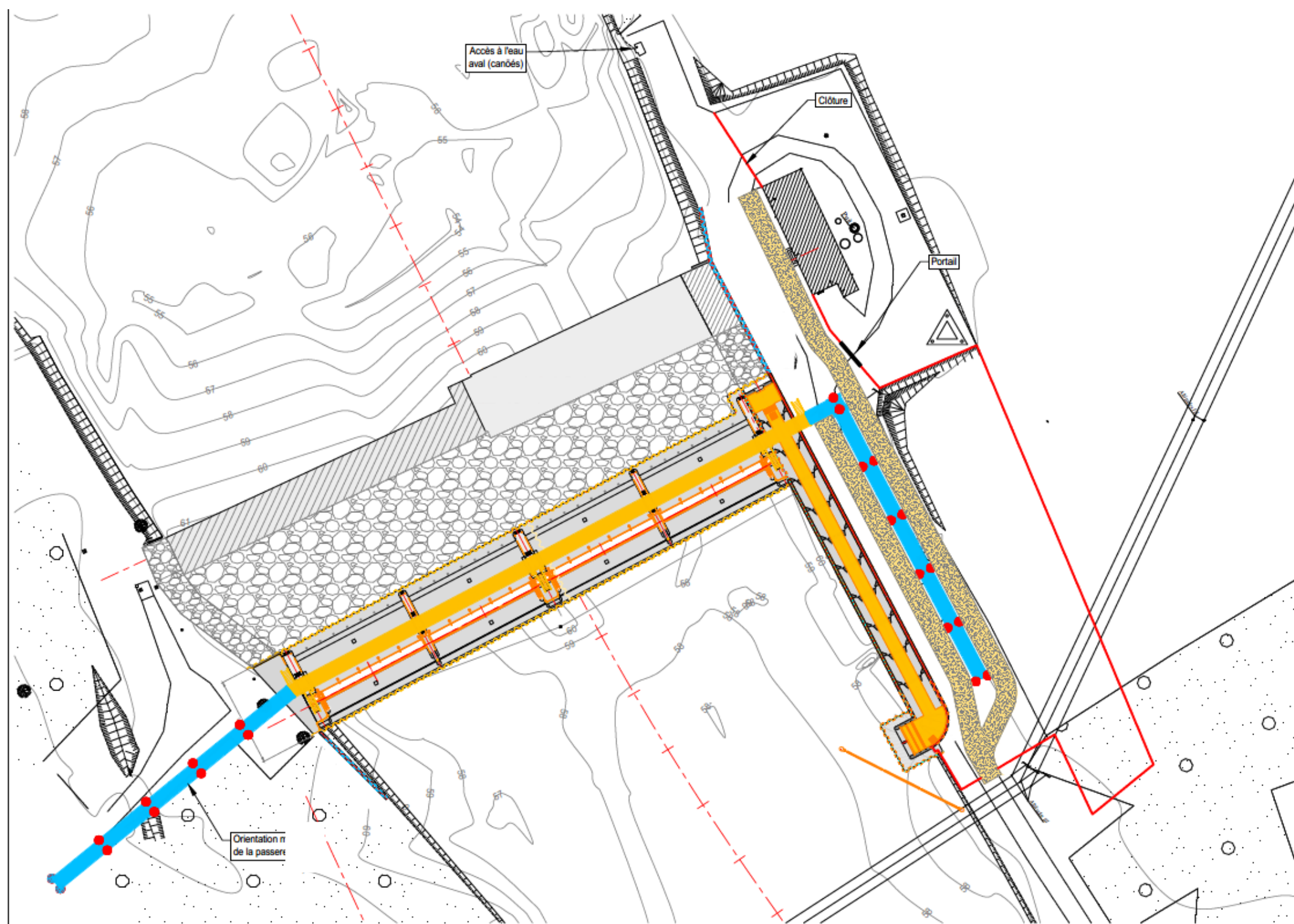
Figure 3. Vue en plan de l'aménagement du nouveau barrage
