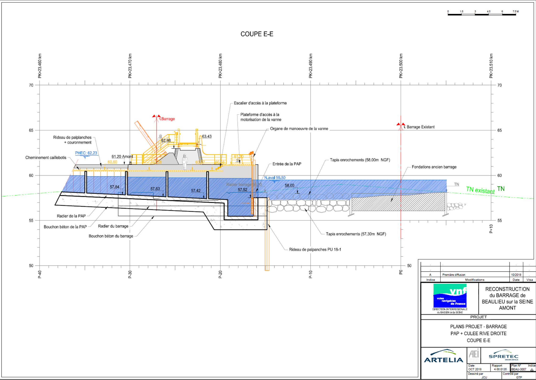
Figure 5. Profil en long du nouveau barrage au droit de la passe à poissons : coupe E-E
