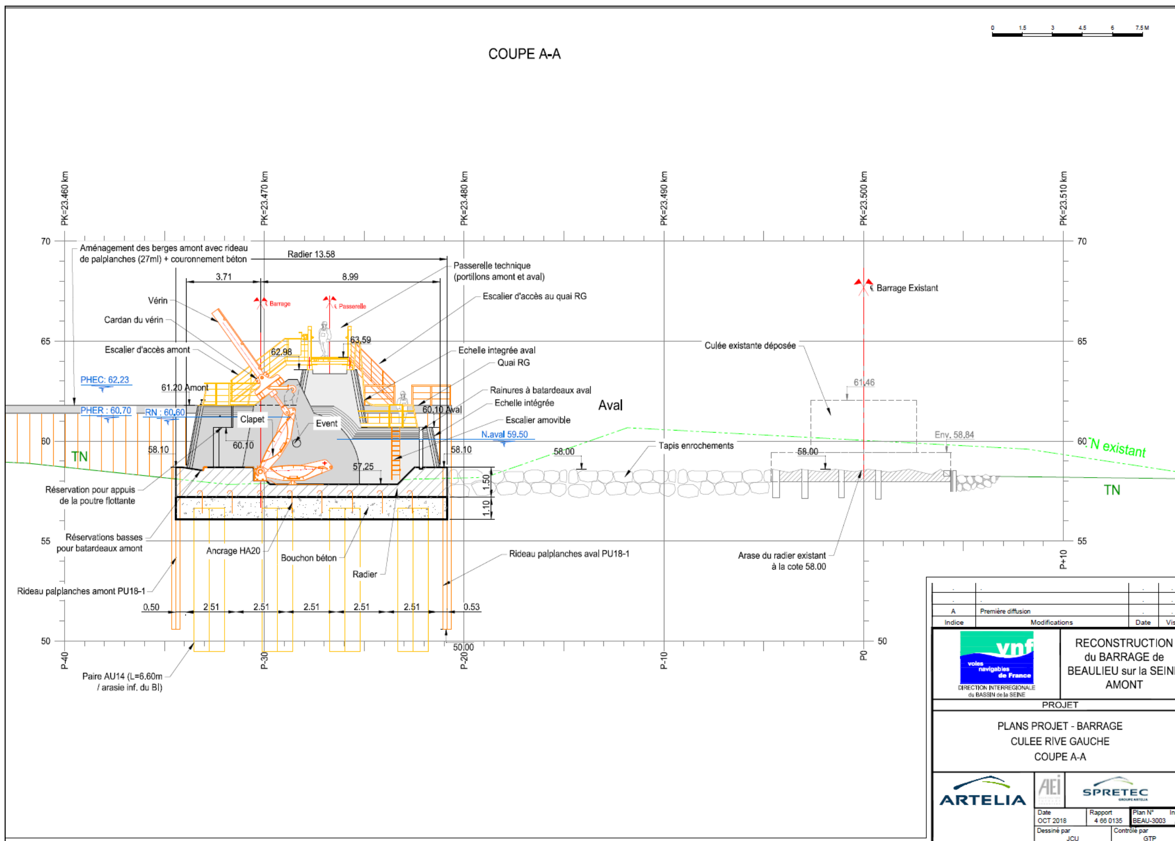
Figure 4. Profil en long du nouveau barrage : coupe A-A
