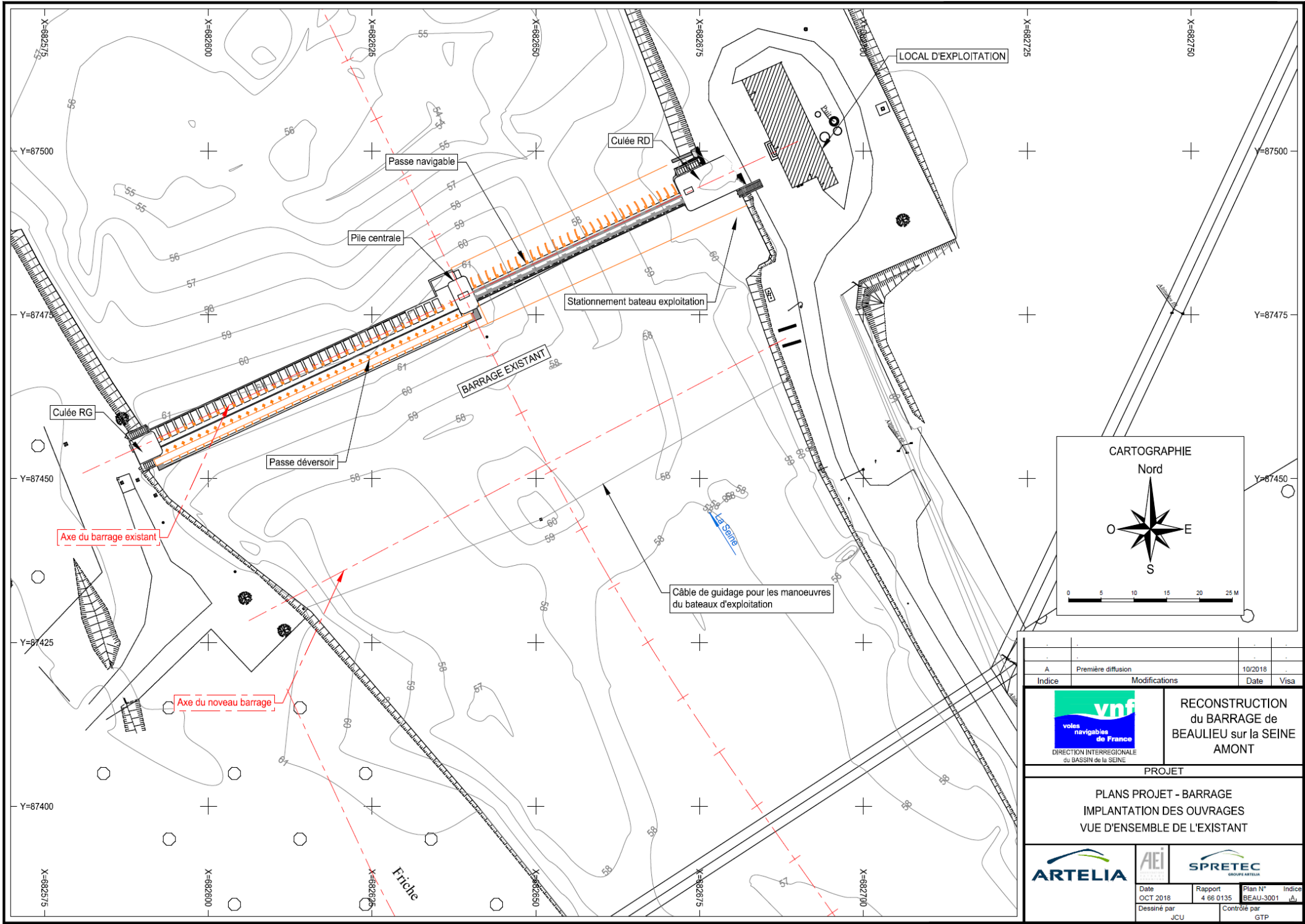
Figure 2. Vue en plan de l'existant
